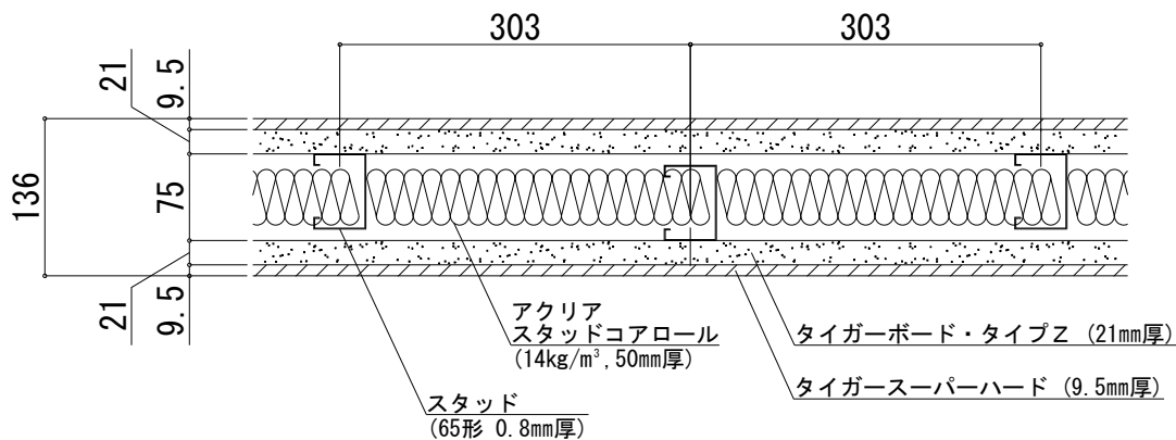
水平断面図（「A-2000・WI アクリア仕様」遮音測定時（S-230-29参照）の壁構造）
