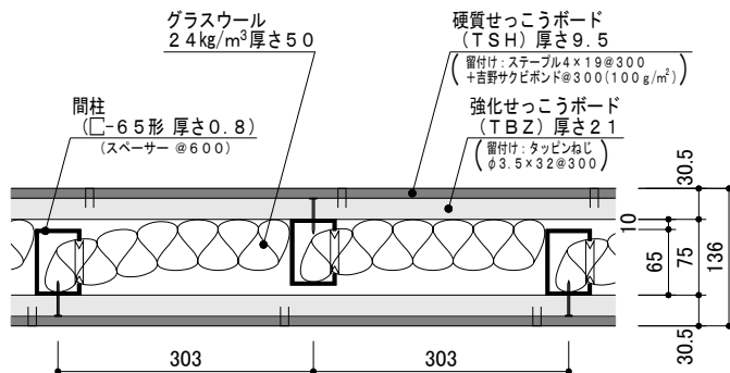
水平断面图
